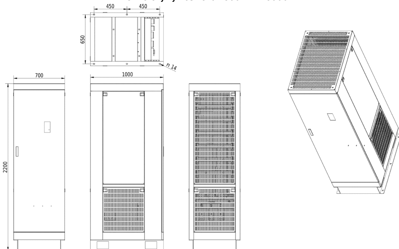
Rozmerový výkres V810 - 800kW 4T8000
