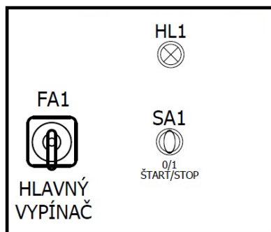
Príklad umiestnenia prvkov na rozvádzači
