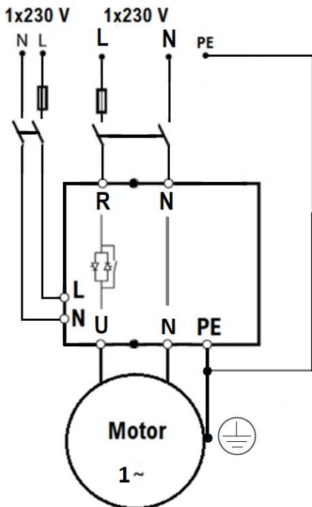
Schéma zapojenia MSS-2S.... silová časť
