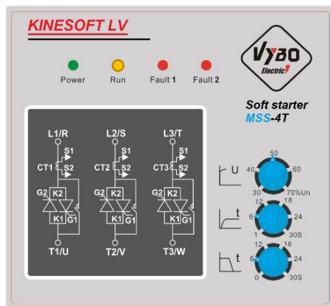
Ovládací panel modelu MSS-4T.....
