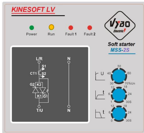
Ovládací panel modelu MSS-2S....
